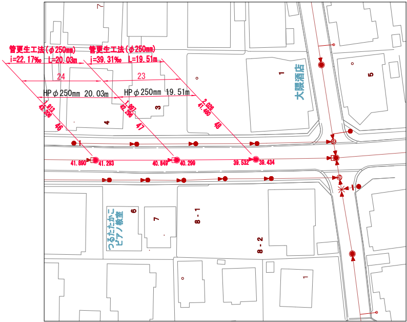
平面図 (1) 縮尺 1/500
