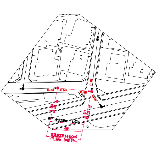
平面図 (2) 縮尺 1/500
