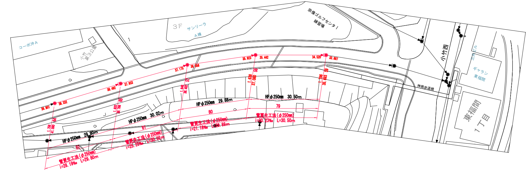
平面図 (1) 縮尺 1/500
