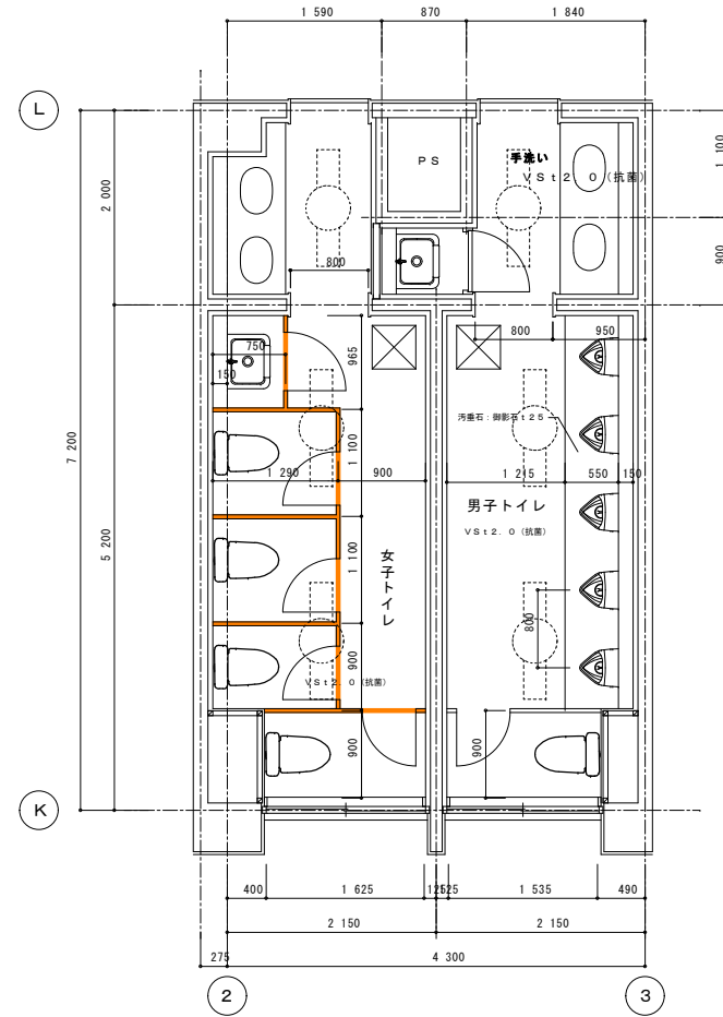
(改修) 平面詳細図
