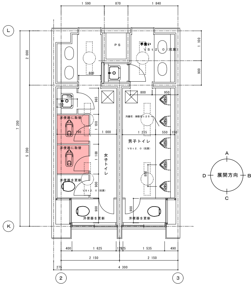
(既存) 平面詳細図
