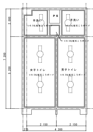
天井伏図 S=1/50
