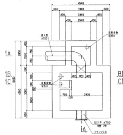
C—C 水平断面图
