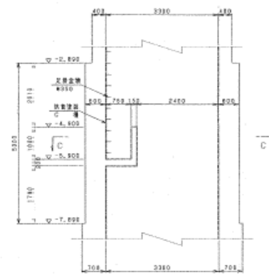
C-C断面図
