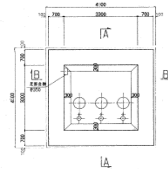
b—b 水平断面图
