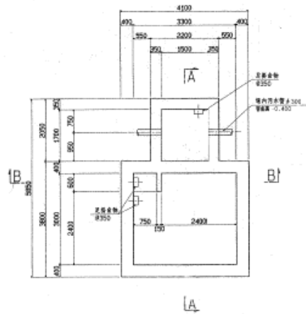
b-b 水平断面图
