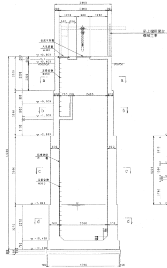
B-B断面図
