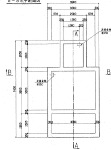
a-a 水平断面图
