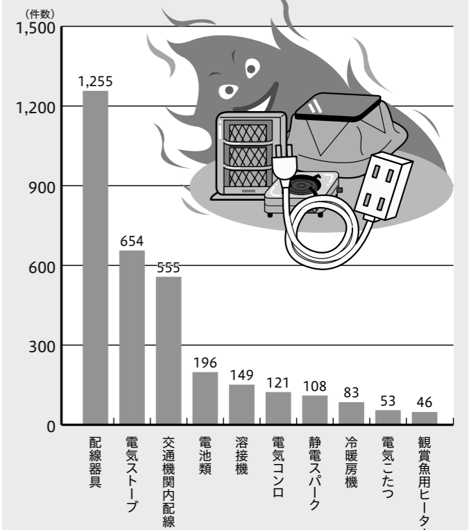
平成23年電気火災の主な発火源 (合計件数3,220件)
