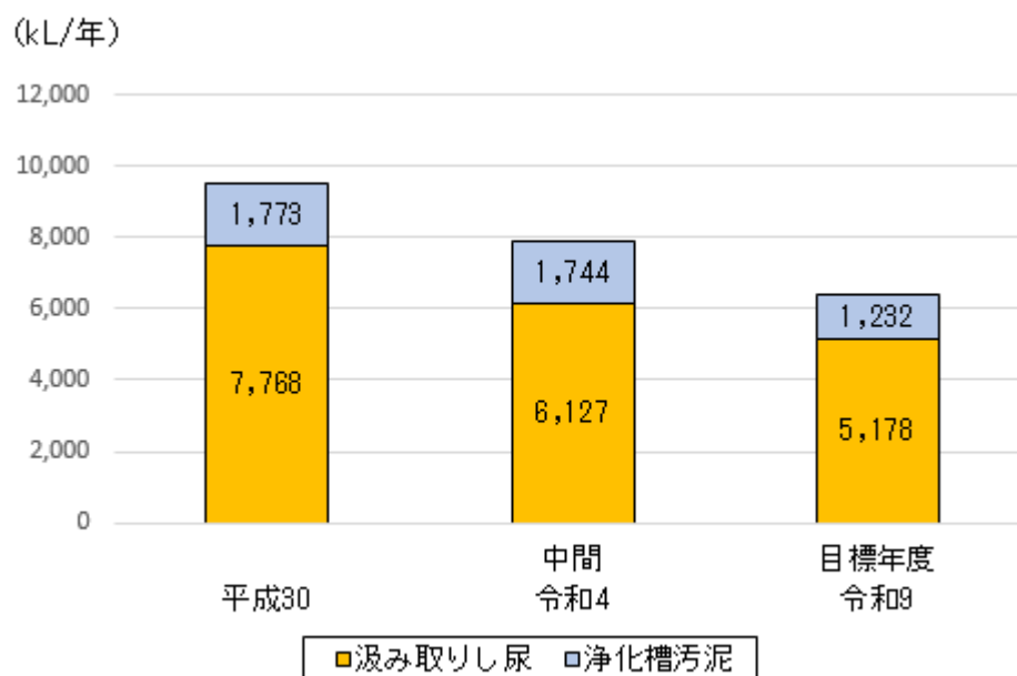
図 7-4 し尿・浄化槽汚泥収集・運搬量の推移
