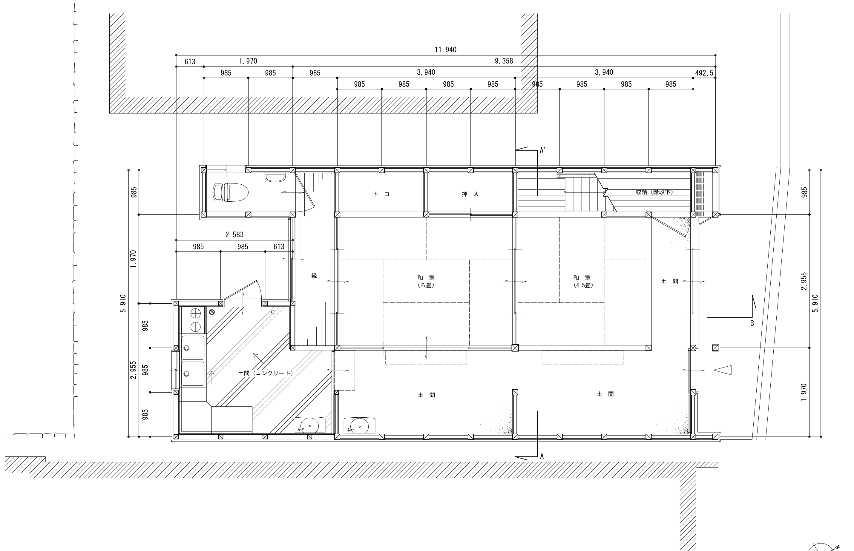
1階平面図
