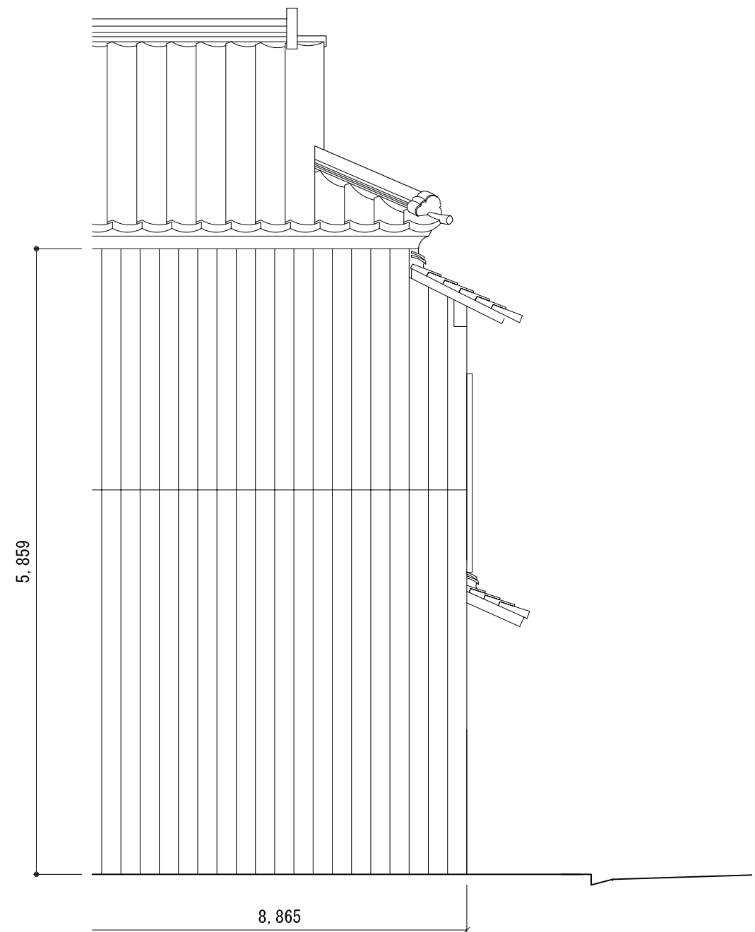
東面立面图
